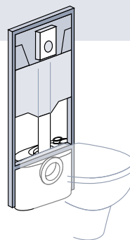
Broyeur intégré au bâti-support Le broyeur est intégré dans un bâti support pré équipé.
